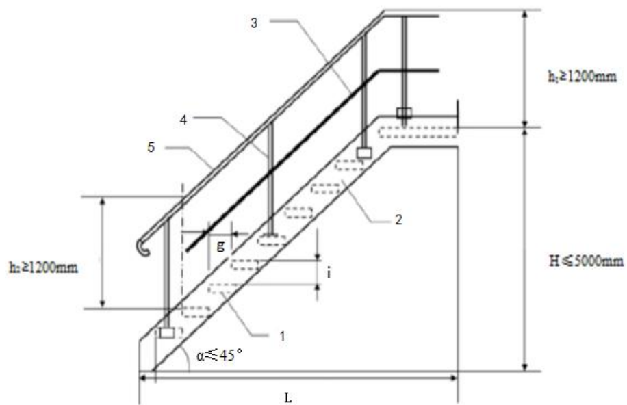
1-踏板;2-梯梁;3-中间栏杆;4-立柱;5-扶手;H-梯高;L-梯跨 h 1 -栏杆高;h 2 -扶手高; \alpha -梯子倾角;i-踏步高;g-踏步宽
